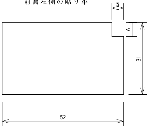
前面左側の貼り革
