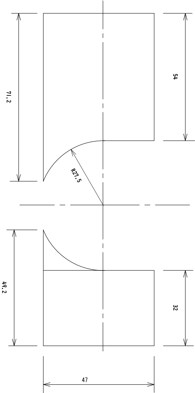
前面の貼り革用型紙
