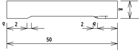
側面の貼り革用型紙
